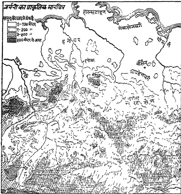
चित्र नं० ४७—जर्मनी का प्राकृतिक मानचित्र
